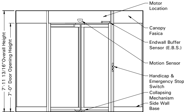
① Elevation
